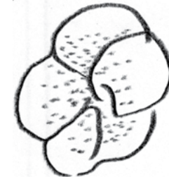
un foraminifère
